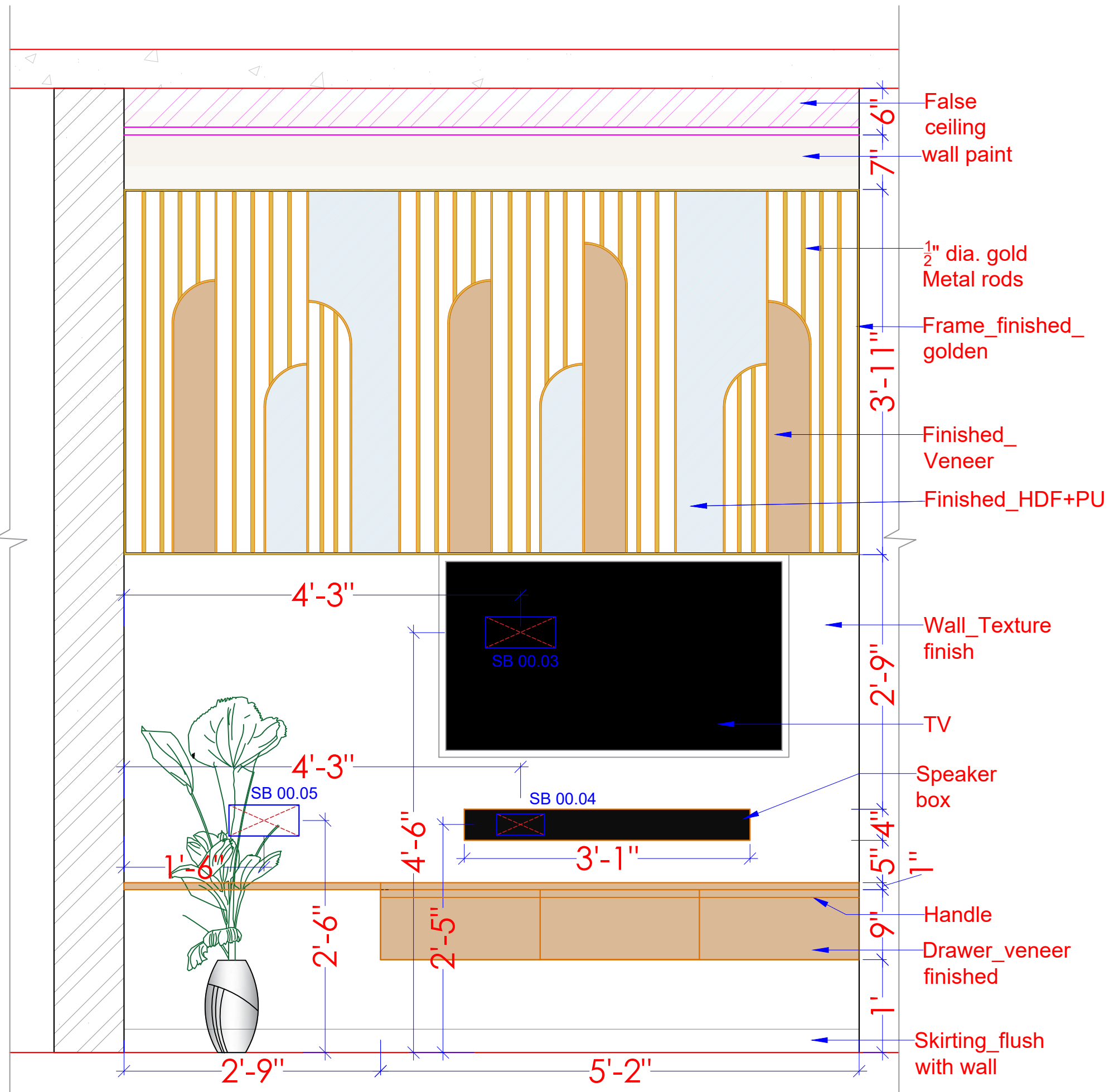
ELEVATION - A
