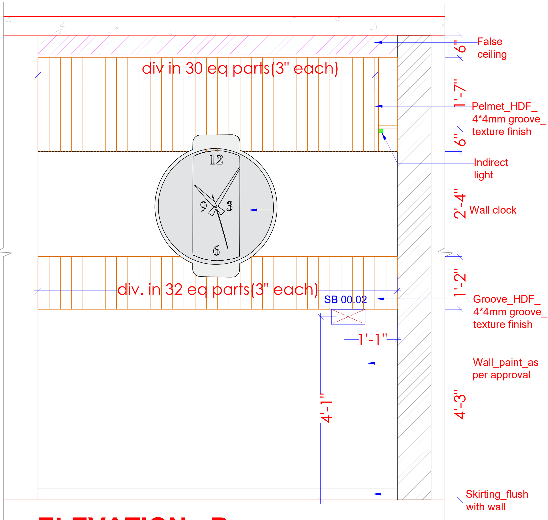
ELEVATION - B
