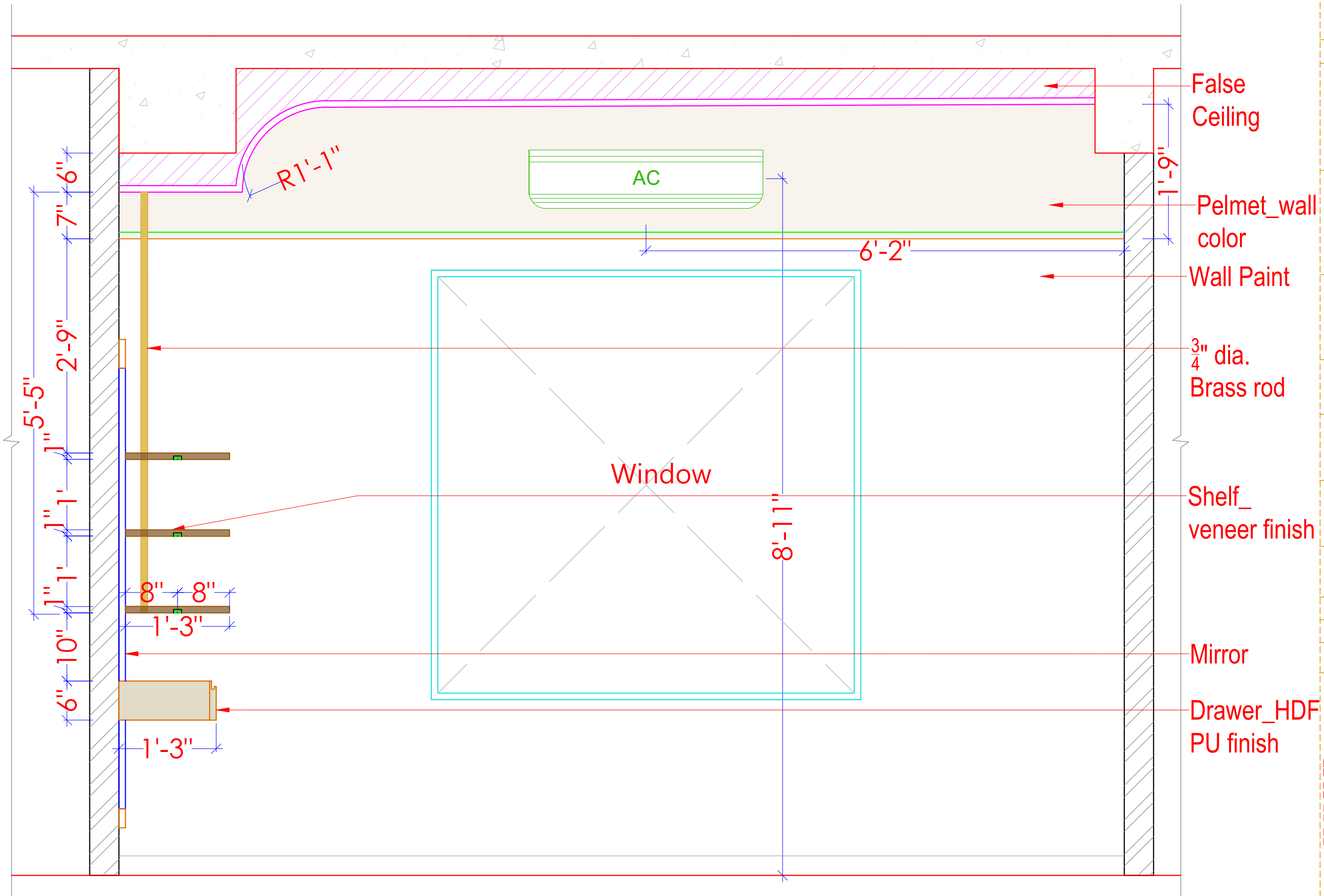
ELEVATION - B
